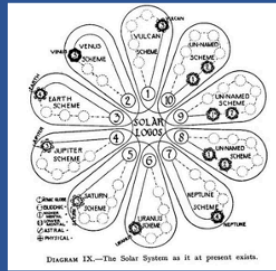
太阳系
