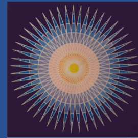
宇宙
